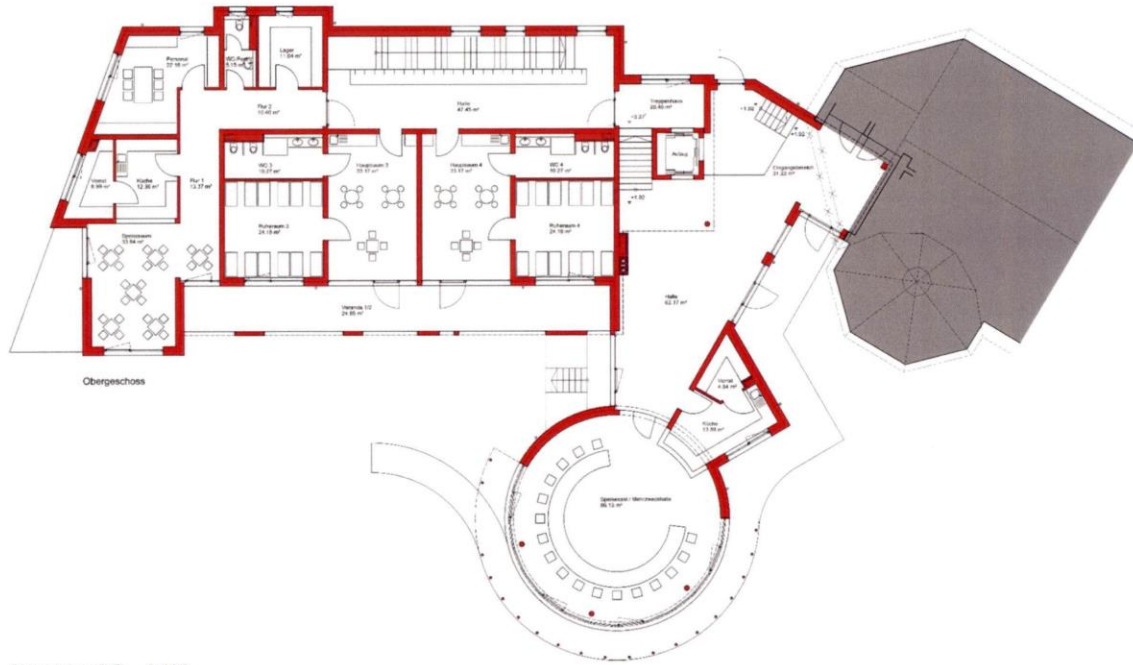
Grundriss OG – 1:100
